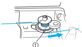
① Fente de guide de la base du bobineur (avec coupe-fil intégré)
